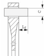
montaje de segmentos rectificadores en cabezas de sujeción L_f = 1,5 C
